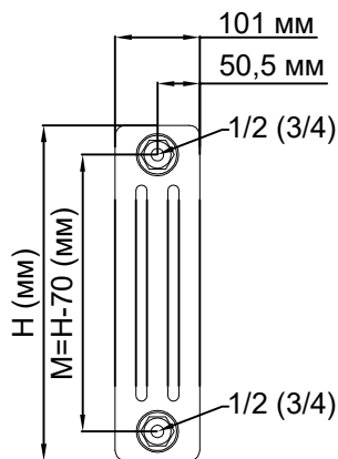
Вид с левого торца
