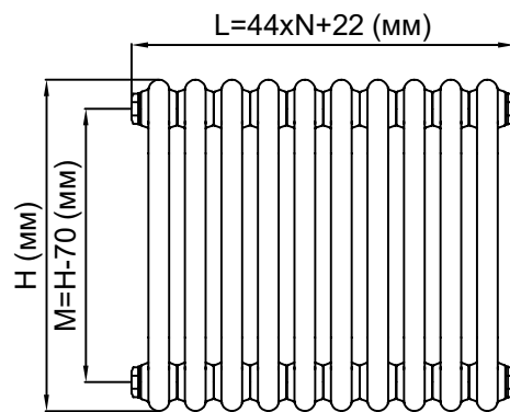
Вид с задней стороны
