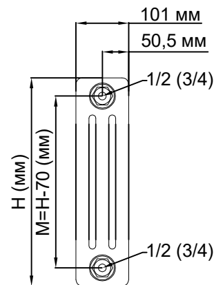
Вид с правого торца
